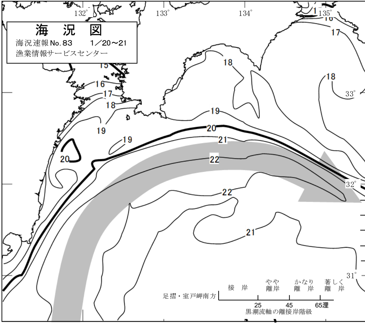
沿岸定点平均 表面水温 (1月15日~1月21日) 数字はセ氏水温
