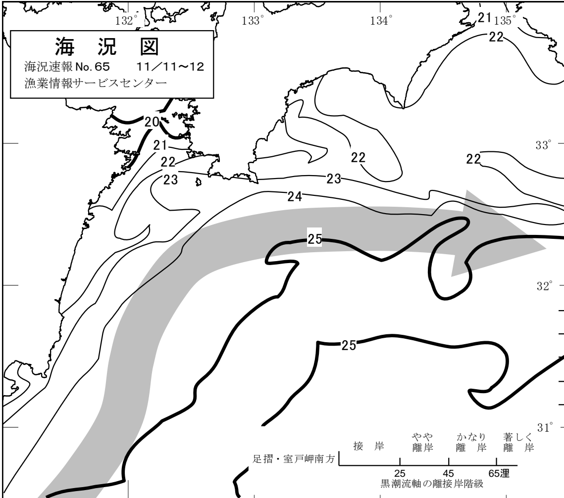
沿岸定点平均 表面水温 (11月6日~11月12日) 数字はセ氏水温
